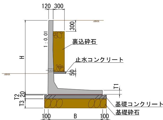
標準施工断面図
